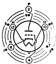
INDEX=LARGE LUG ●=PIN CUT OFF 12AQ
